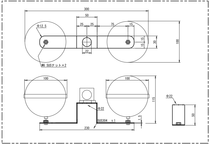
PROWEI PRO-F(SUS架台型)吸い込みフロート付き外形図
