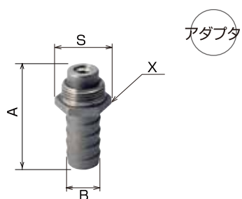
VDF アダプタ付 寸法表 (単位 : mm)
